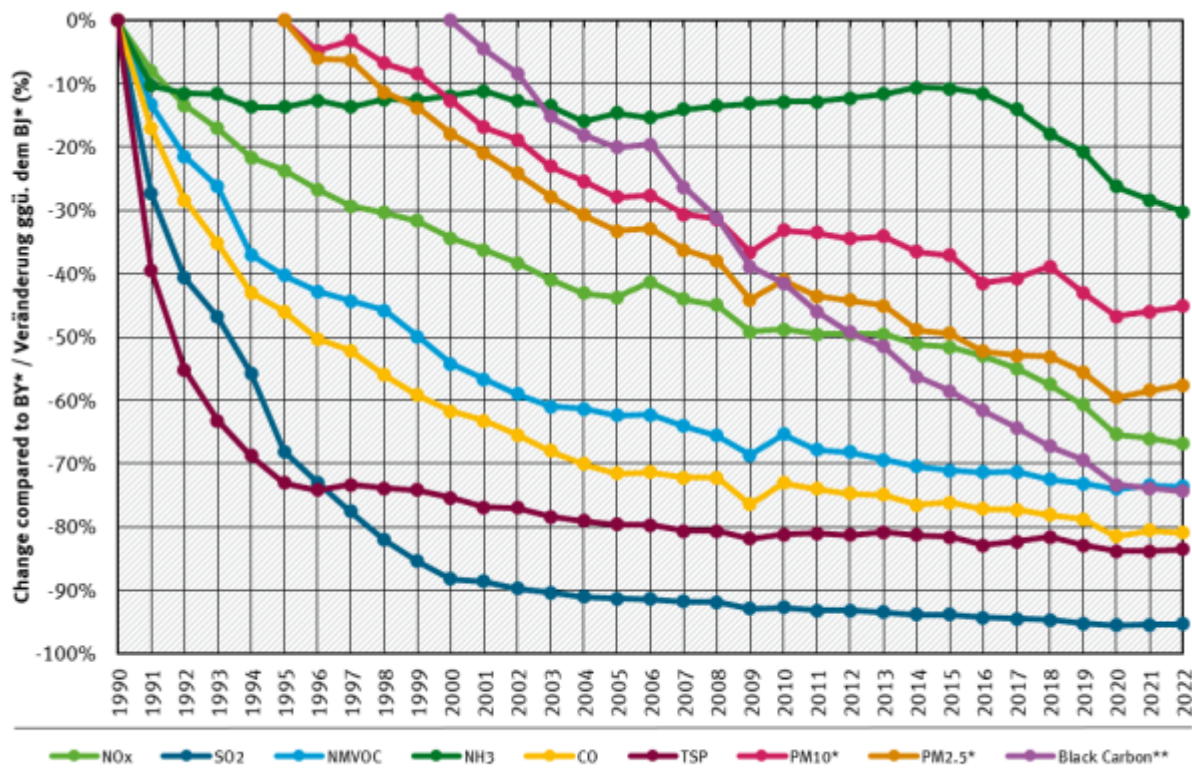
* Base Year (BY) 1990, 1995 for PM10/PM2.5 / Basisjahr (BJ) 1990, 1995 für Feinstaub ** Black Carbon emissions: from 2000 / Black Carbon Emissionen erst ab 2000 Quelle: German Emission Inventory (15.03.2024)
