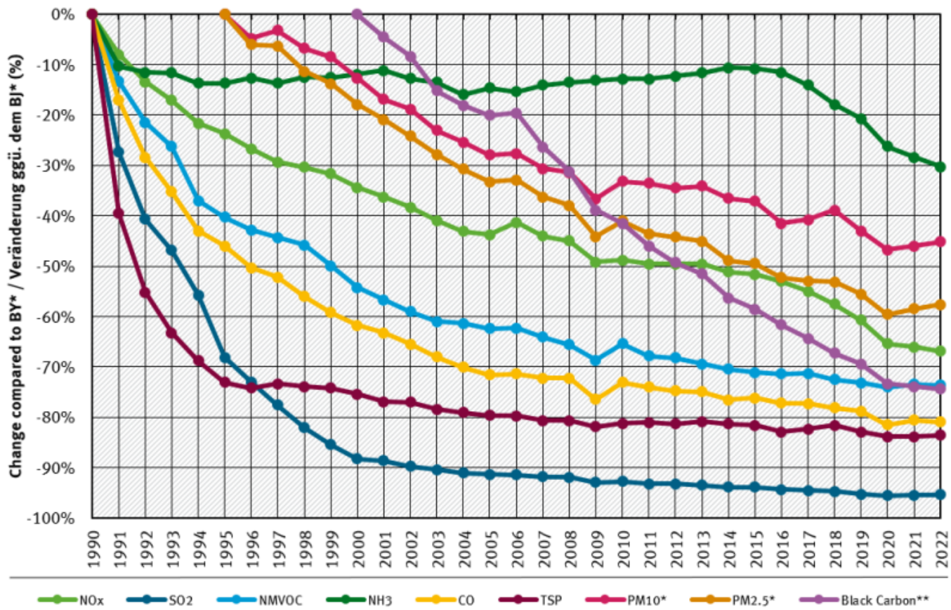
* Base Year (BY) 1990, 1995 for PM10/PM2.5 / Basisjahr (BJ) 1990, 1995 für Feinstaub ** Black Carbon emissions from 2000 / Black Carbon Emissionen erst ab 2000 Quelle: German Emission Inventory (15.03.2024)
